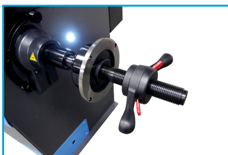
WSKAŹNIK LASEROWY ORAZ OŚWIETLENIE WNĘTRZA KOŁA
