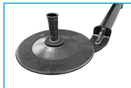
TALERZ RAMIENIA POMOCNICZEGO WSPOMAGAJĄCY MONTAŻ/DEMONTAŻ OPONY
