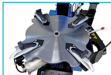
PROFILOWANY STÓŁ Z WYTRZYMAŁEJ STALI
